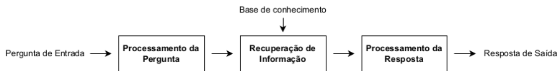
Figura 18.2: Arquitetura geral de um sistema de QA.
